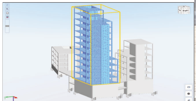
SOFiSTiK Erdbebenberechnung / Seismic Analysis
